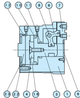
CKA-20AS 標準タイプ
