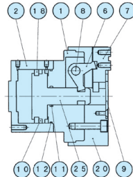
CKA-50MS ~ 70MS 標準タイプ
