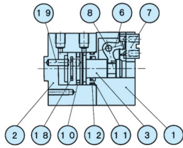
CKA-15AS 標準タイプ
