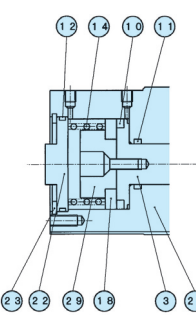
CKA-20AS NO タイプ
