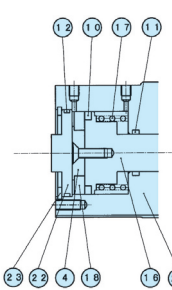
CKA-20AS NC タイプ
