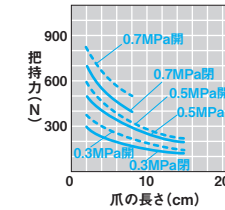
■CKA・CKB・CKD-40AS
