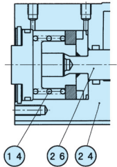
CKA-50MS ~ 70MS NO タイプ
