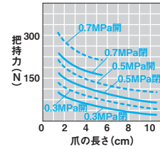
■CKA・CKB・CKD-30AS
