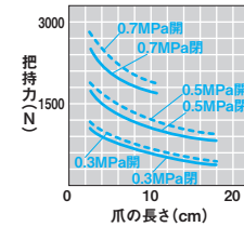
■CKA・CKB・CKD-70MS
