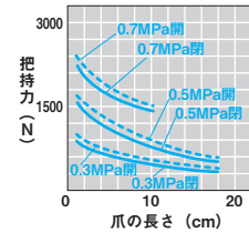
■CKA・CKB・CKD-60MS
