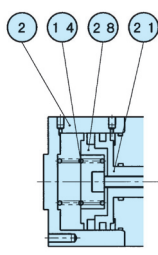
CKA-50MS ~ 70MS NO タイプ
