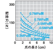
■CKA・CKB・CKD-25AS
